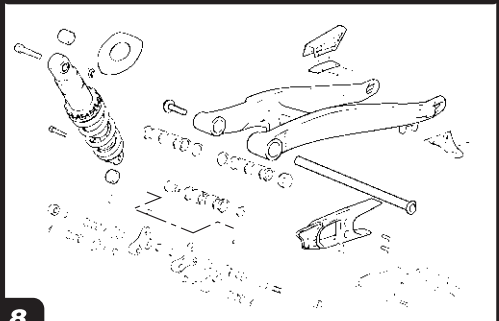
Basculante / Swingarm CASCAS TXT PRO 06
